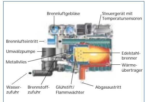
Wasserheizgerät Thermo Top C
