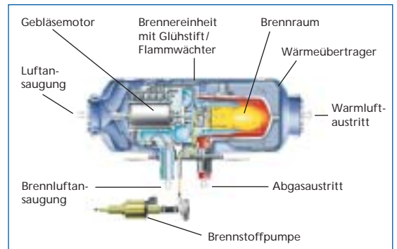
Luftheizgerät Air Top 2000 S
